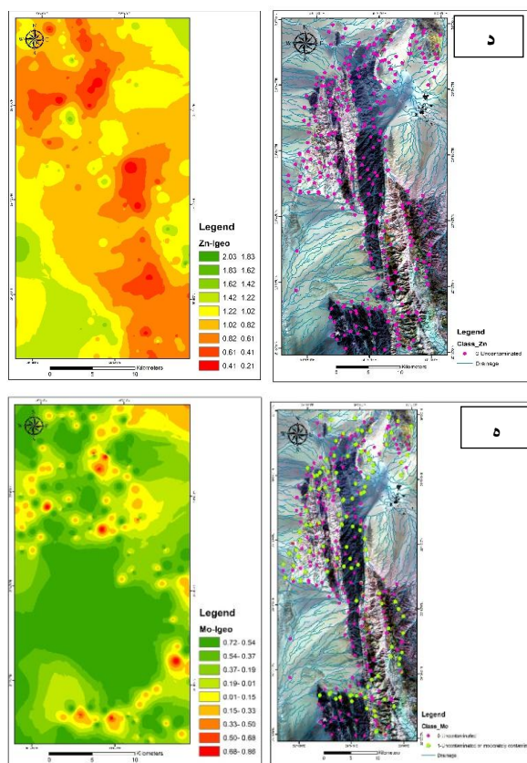
شکل ۱۱. پراکنش مکانی شاخص زمین‌انباشتگی (د) روی و (ه) مولیبدن در خاک سطحی منطقه نصرت‌آباد
