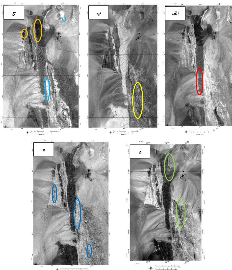
شکل ۲. (الف) نسبت بانندی ۴/۷، سنگ‌های غنی از تالک و سرپانتینیت (هدف: پیکسل‌های روشن)؛ (ب) نسبت بانندی ۲/۴، سنگ‌های گرانیتوئیدی (هدف: پیکسل‌های روشن) و آمفیبولیت‌ها و افیولیت‌های بسیاربریده‌شده (هدف: پیکسل‌های خاکستری تیره تا سیاه)؛ (ج) نسبت بانندی ۶/۸، متاولکانیک‌ها، گابرو - دیوریت‌ها (هدف: پیکسل‌های خاکستری) و گرانیتوئیدهای نفوذی (هدف: پیکسل‌های خاکستری تیره تا سیاه) و سنگ‌های غنی از آهن (الترامافیک - مافیک) (هدف: پیکسل‌های روشن)؛ (د) نسبت بانندی ۴/۱، گرانودیوریت‌ها و سیانوگرانیت‌ها (هدف: پیکسل‌های خاکستری تیره)؛ (ه) نسبت بانندی ۴/۳ × ۲/۳، سنگ‌های حاوی کوارتز - دیوریت و متاولکانیکی (هدف: پیکسل‌های خاکستری روشن)
