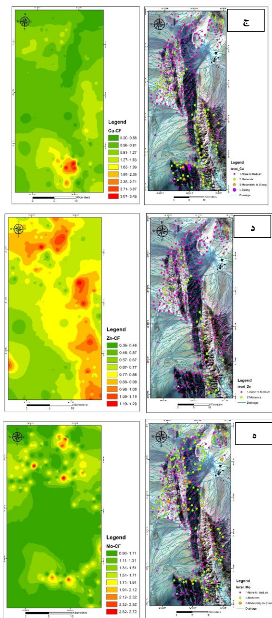
شکل ۱۳. پراکنش مکانی ضریب آلودگی (ج) مس، (د) روی، و (ه) مولیبدن در خاک سطحی منطقه نصرت آباد
