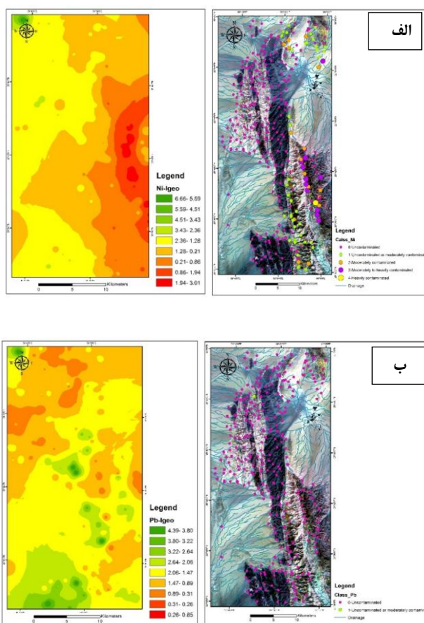
شکل ۱۰. پراکنش مکانی شاخص زمین‌انباشتگی (الف) نیکل، (ب) سرب، (ج) مس در خاک سطحی منطقه نصرت‌آباد
