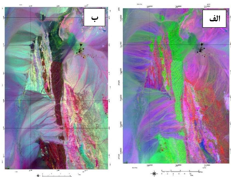
شکل ۳. تصاویر حاصل از ترکیب رنگی کاذب ۳ باند مختلف (قرمز، سبز، آبی): (الف) R: 4/7, G: 2/4, B: 6/8 و (ب) R: 4/7, G: 4/1, B: 2/3 \times 4/3
