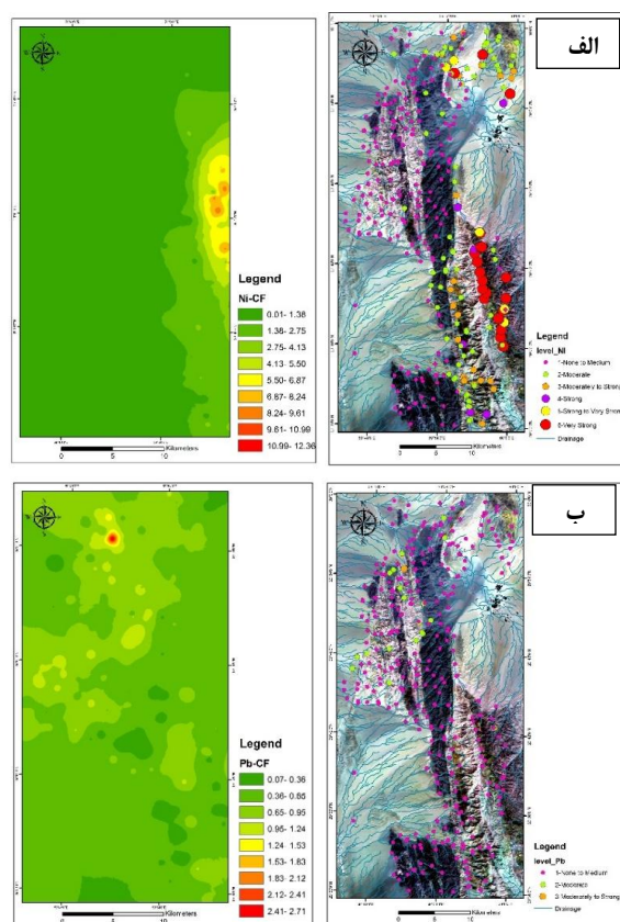
شکل ۱۲. پراکنش مکانی ضریب آلودگی (الف) نیکل و (ب) سرب در خاک سطحی منطقه نصرت آباد
