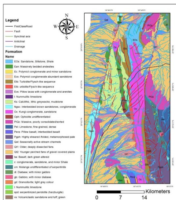
شکل ۱. موقعیت و نقشه زمین‌شناسی منطقه ناصرت آباد
