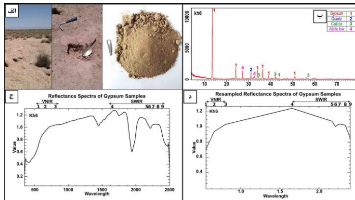
شکل ۱۰. نمونه ژیبس مربوط به کفه خاتون‌آباد. الف) نمایی از کفه خاتون‌آباد و نمونه ژیبس مورد استفاده در طیف‌نگاری، ب) نمودار XRD نمونه ژیبس کفه خاتون‌آباد، ج) منحنی طیفی نمونه ژیبس، د) منحنی طیفی بازنویسی شده نسبت به باندهای استر نمونه ژیبس خاتون‌آباد
