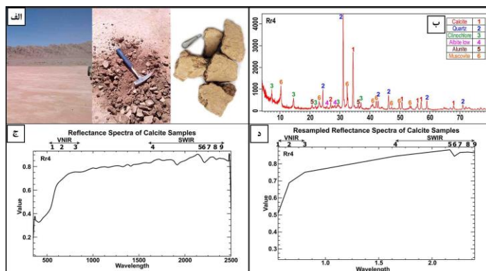
شکل ۱۲. نمونه کلسیت مربوط به منطقه راور. الف) نمایی از کالکریت و نمونه برداشت شده برای طیف نگاری، ب) طیف XRD نمونه شکل الف، ج) منحنی طیفی کلسیت، د) منحنی طیفی کلسیت بازنویسی شده نسبت به باندهای استر
