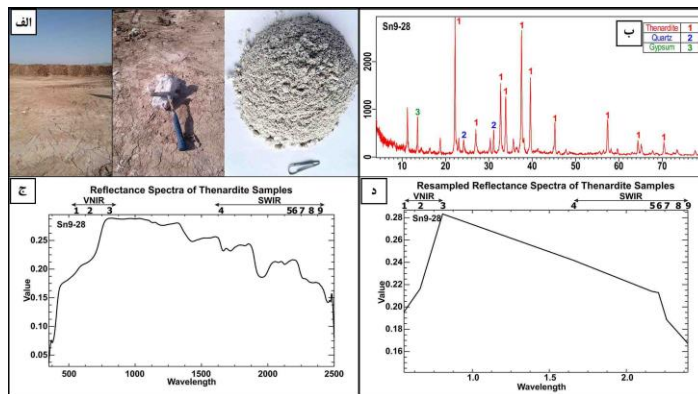
شکل ۱۱. نمونه تناردیت مربوط به جنوب شرقی کفه نمکی سیرجان. الف) نمایی از منطقه تناردیت‌دار و نمونه برداشت شده برای طیف‌نگاری، ب) طیف XRD نمونه شکل الف، ج) منحنی طیفی تناردیت، د) منحنی طیفی تناردیت بازنویسی شده نسبت به باندهای استر
