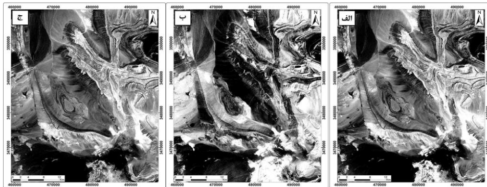
شکل ۷. بارزسازی کانی‌های تبحیری منطقه راور با استفاده از روش CEM. الف) هالیت، ب) ژپس، و ج) کلسیت
