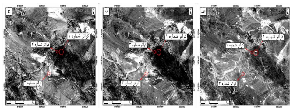
شکل ۸. بارزسازی کانی‌های تبحیری منطقه راین با استفاده از روش CEM. الف) هالیت، ب) تنداردیت، و ج) کلسیم
