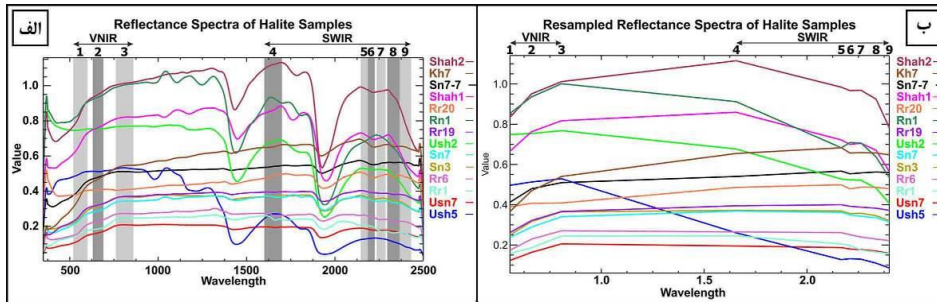
شکل ۱. الف) طیف نمونه‌های هالیت، نوارهای خاکستری رنگ، پهنای باندهای سنجنده استر روی طیف الکترومغناطیس را نشان می‌دهد. ب) طیف‌های نمونه‌های هالیت بازنویسی شده بر اساس باندهای سنجنده استر
