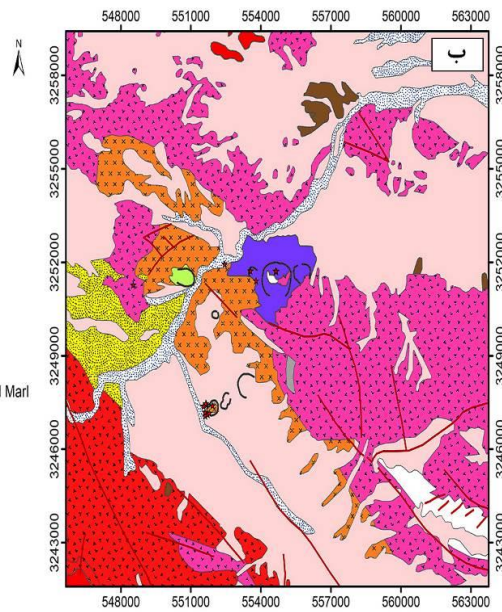
شکل ۳. الف) نقشه زمین‌شناسی منطقه مطالعاتی کَشکوتیه (ناظم‌زاده شعاعی و عزیزان، ۱۳۵۲)، ب) نقشه زمین‌شناسی منطقه مطالعاتی رابن (جوکوویچ و حالویاتی، ۱۹۷۲)
