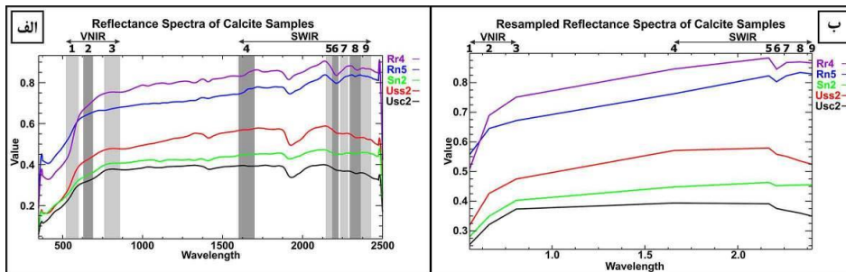
شکل ۴. الف) طیف نمونه‌های کلسیت، نوارهای خاکستری رنگ پهنای باندهای سنجنده استر روی طیف الکترومغناطیس را نشان می‌دهد. ب) طیف‌های نمونه‌های کلسیت بازنویسی شده بر اساس باندهای سنجنده استر
