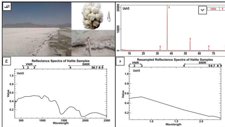
شکل ۹. هالیت خالص مربوط به کفه نمکی سیرجان. الف) نمایی از کفه نمکی سیرجان به همراه نمونه برداشت شده برای طیف‌نگاری. ب) بافت گل‌کلمی نمونه هالیت در عکس مشهود است، ب) نمودار XRD نمونه، ج) منحنی طیف نمونه نمک خالص برداشت شده از کفه نمکی سیرجان، د) منحنی طیفی بازنویسی شده نسبت به باندهای استر نمونه هالیت کفه نمکی سیرجان
