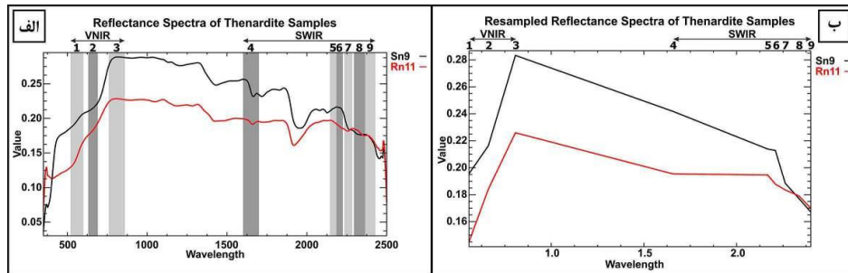
شکل ۳. الف) طیف نمونه‌های تناردیت، نوارهای خاکستری رنگ پهنای باندهای سنجنده استر روی طیف الکترومغناطیس را نشان می‌دهد. ب) طیف‌های نمونه‌های تناردیت بازنویسی شده بر اساس باندهای سنجنده استر
