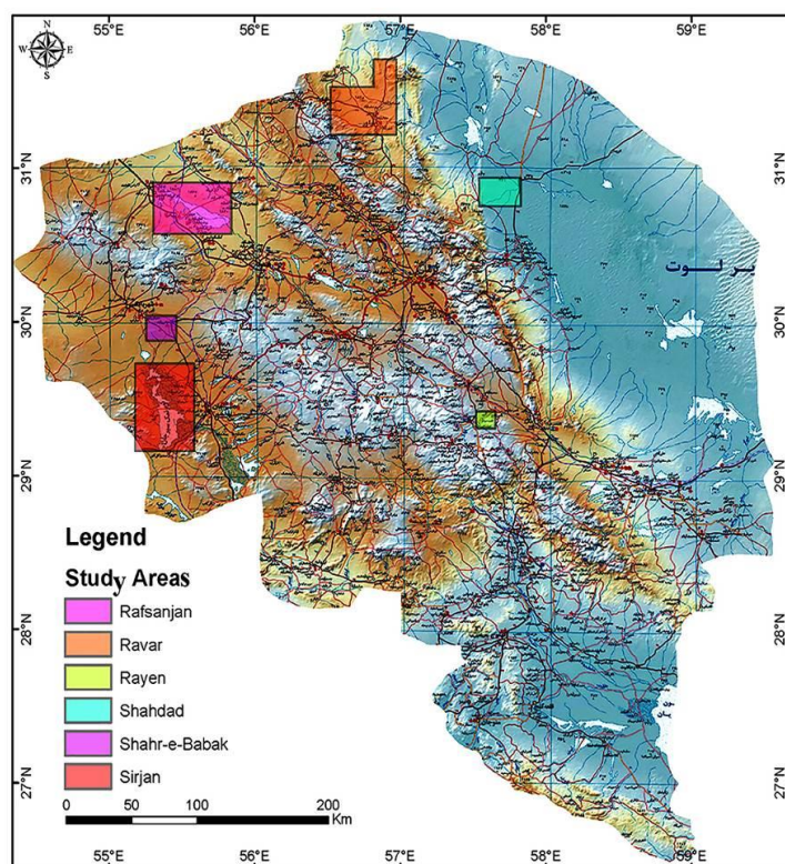
شکل ۵. راه‌های دسترسی به مناطق مورد مطالعه (نقشه راه‌های ایران، انتشارات گیتاژ، ۱۳۸۷)
