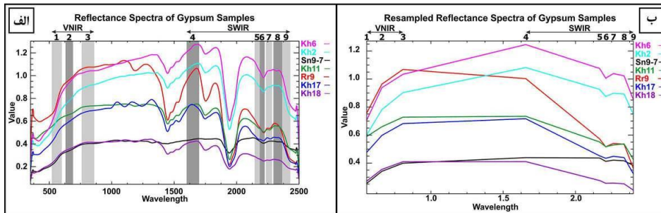
شکل ۲. الف) طیف نمونه‌های گیپس، نوارهای خاکستری رنگ، پهنای باندهای سنجنده استر روی طیف الکترومغناطیس را نشان می‌دهد. ب) طیف‌های نمونه‌های گیپس بازنویسی شده بر اساس باندهای سنجنده استر
