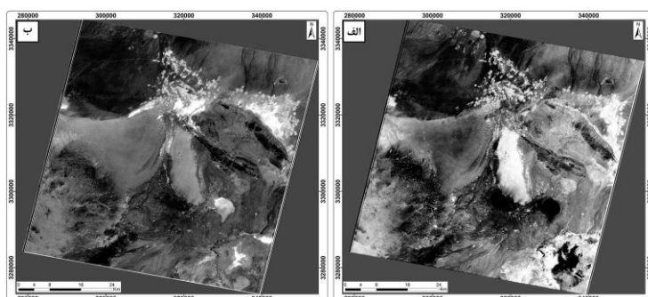
شکل ۶. بارزسازی کانی‌های تبخیری منطقه شهربابک با استفاده از روش CEM. الف) هالیت، ب) ژپس
