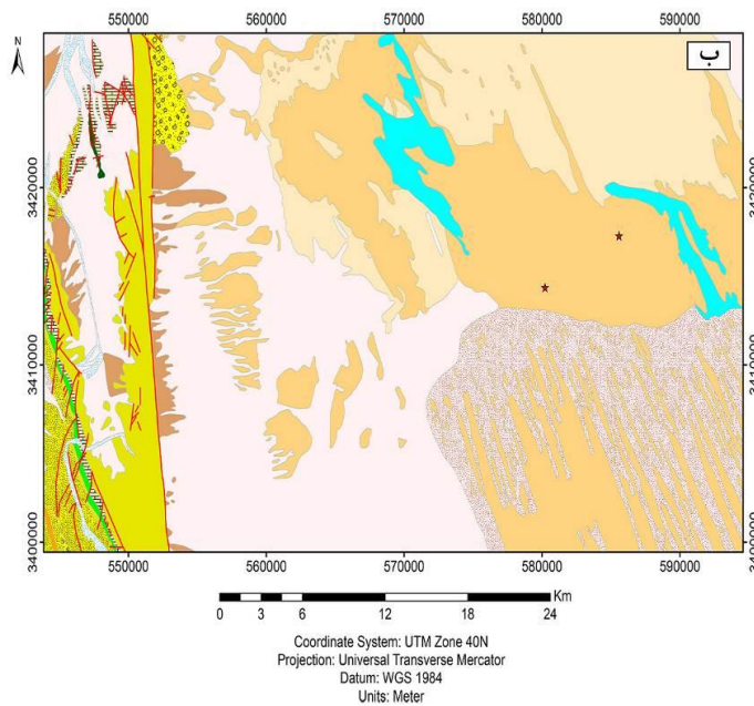
شکل ۴. الف) نقشه زمین شناسی منطقه مطالعاتی خاتون آباد (سردیک و همکاران، ۱۹۷۱)، ب) نقشه زمین شناسی منطقه مطالعاتی شهداد (سهندی، ۱۳۷۴)
