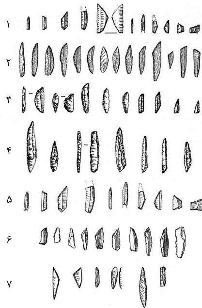
تصویر ۳. میکرولیت‌های هندسی و ریز تیغه‌های کولدار و قطع شده شاخص صنعت زرزی (۱. غار خر؛ ۲. زرزی؛ ۳ و ۴. ورواسی؛ ۵. مرگورگلان سراب؛ ۶. شنیدر؛ ۷. پاسنگر). مقیاس‌ها متفاوت است (Garrod 1930; Hole 1970; Mortensen 1993; Olszewski 1993b; Smith 1986; Solecki 1964)
