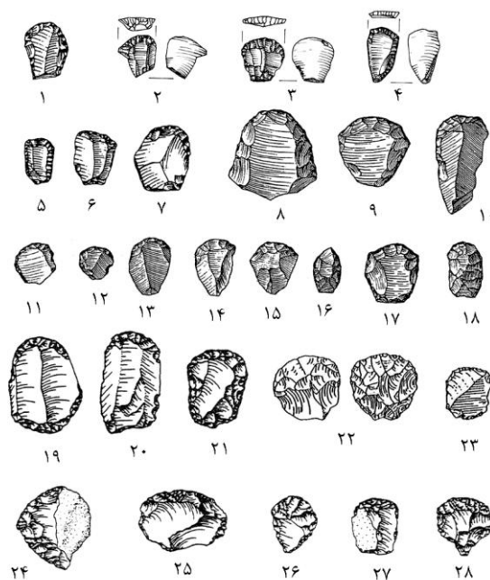
تصویر ۵. خراشنده‌ها در صنعت زرزنی (۱ و ۵ - ۷. غار خر؛ ۲ - ۴. مرروز؛ ۸ - ۱۸. زرزنی؛ ۱۹ - ۲۱ و ۲۴ - ۲۸. ورواسی؛ ۲۲ - ۲۳. پاسنگر) (Garrod 1930; Hole 1970; Mortensen 1993; Olszewski 1993b; Smith 1986)
