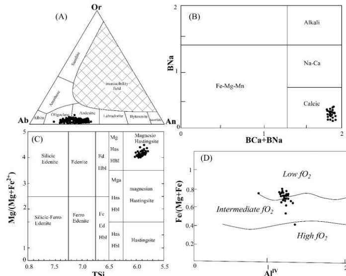
شکل ۶. (A) ترکیب پلاژیوکلازهای سنگ‌های دایک آندزیتی منطقه حسن‌آباد در نمودار مثلثی Or-Ab-An (دیر و همکاران ۱۹۹۲). پلاژیوکلازهای دایک آندزیتی منطقه در محدوده الیگوکلاز-آندزین قرار دارند؛ (B) نمودار رده‌بندی آمفیبول‌ها (لیک و همکاران ۱۹۹۷) بر اساس BNa در برابر BCa + BNa. موقعیت نمونه‌های مورد مطالعه در محدوده کلسیک است؛ (C) نمودار رده‌بندی آمفیبول‌ها بر اساس Mg/(Mg+Fe 2+ ) در برابر TSi (لیک و همکاران ۱۹۹۷). موقعیت نمونه‌های مورد مطالعه در محدوده مگنزیو هاستینگزیت است؛ (D) ارزیابی فوگاسیتته اکسیژن با استفاده از ترکیب شیمیایی آمفیبول‌ها (اندرسون و اسمیت ۱۹۹۵) برای زینولیت‌های موجود در سنگ‌های خروجی منطقه حسن‌آباد
