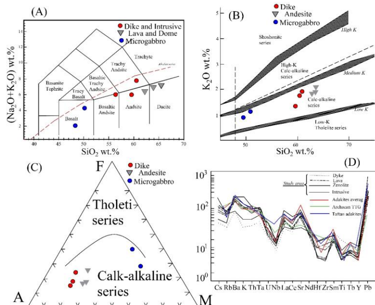
شکل ۴. (A) نمودار نام‌گذاری سنگ‌های خروجی مجموع آکالن در مقابل سیلیس برای سنگ‌های خروجی (لوباس و همکاران ۱۹۸۶)؛ (B) موقعیت نمونه‌ها در نمودار پکسریلو و تایلور (۱۹۷۶) بر حسب تغییرات K_2O در برابر SiO_2 ؛ (C) نمودار AFM جهت تعیین سری ماگمایی (اروین و باراگار ۱۹۷۱)؛ (D) نمودار عنکبوتی به‌هنجار شده در برابر ترکیب متوسط گوشته‌ای (سان و مک دونالد ۱۹۸۹)
