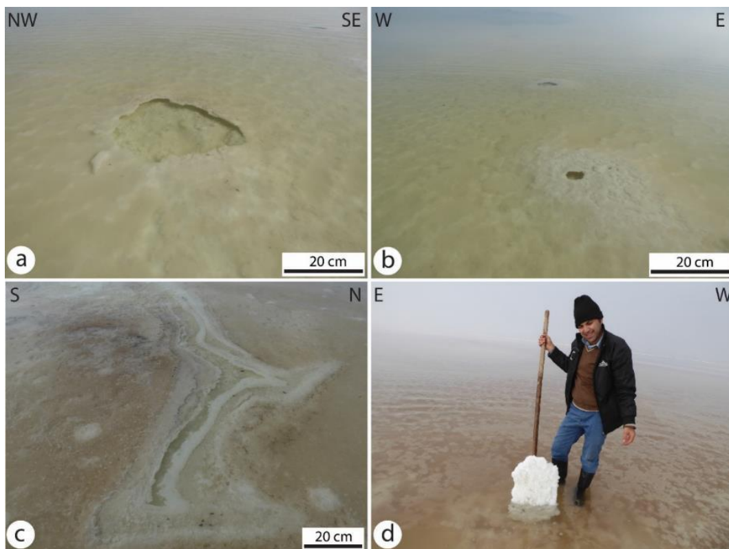
شکل ۶. (a) ساخت‌های انحلالی ژئودمانند حاصل از انحلال نمک بستر دریاچه توسط آب شیرین؛ (b و c) تبخیر شورابه و بسته شدن سطح حفره‌ها توسط رشد بلورهای هالیت و نهایتاً رشد و تشکیل کریستال‌های بزرگ سیلویت در داخل حفره‌ها؛ (d) نمونه‌ای از کانی‌های درشت‌بلور سیلویت تشکیل شده در داخل حفره‌های ژئودمانند.
