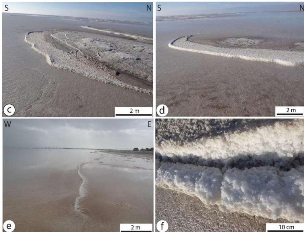
ادامه شکل ۱. (a و b و c و d) مراحل تشکیل ساخت نمکی نعل اسبی با دیواره مرتفع و قائم به سمت دریا و بخش کم ارتفاع و کم شیب به سمت ساحل در سواحل باختری و شمال باختری دریاچه؛ (f) رشد بلورهای درشت هالیت در بخش مرتفع ساخت های موجی شکل.
