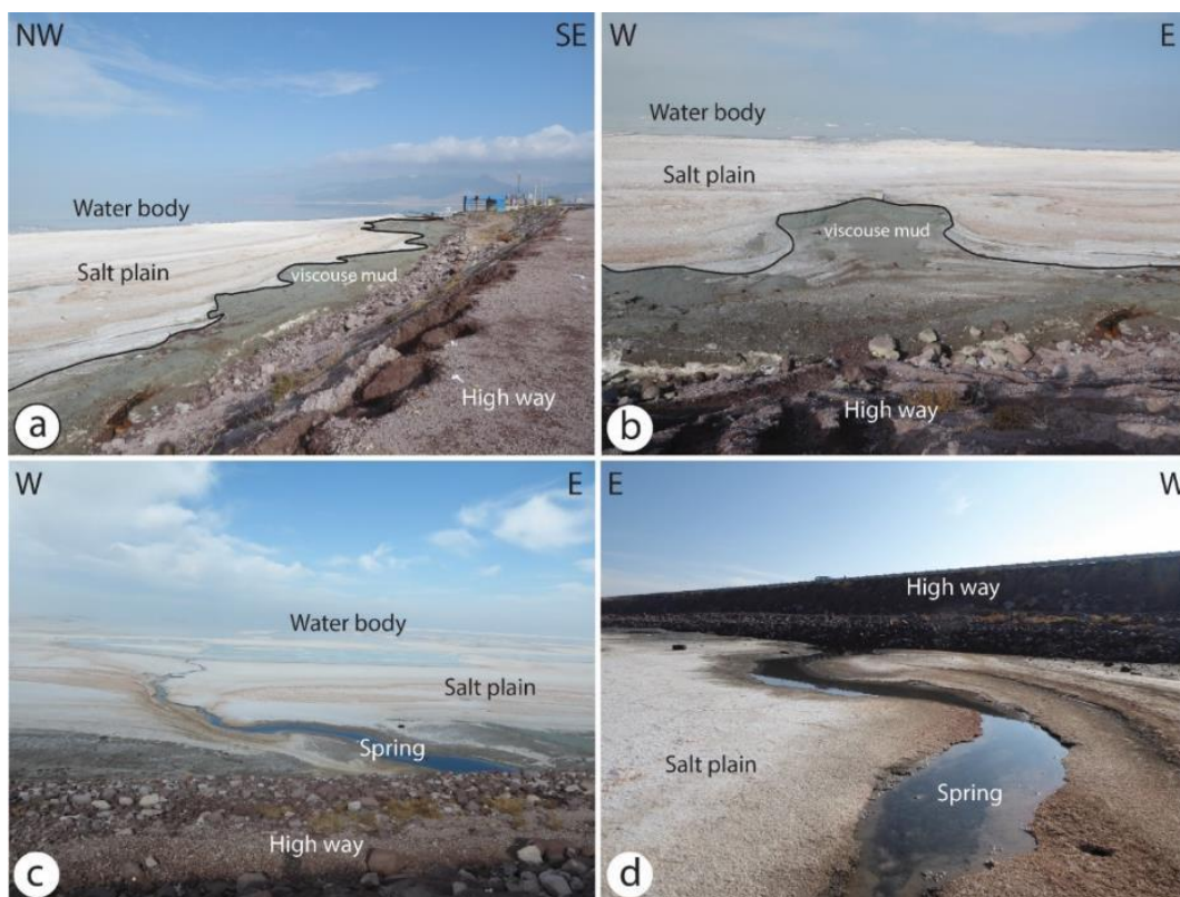
شکل ۱۴. روان‌گرایی گل‌های بستر دریاچه با حالت سینوسی در حاشیه شمالی و جنوبی میان‌گذر شهید کلاتری؛ (a و b) روان‌گرایی گل‌های بستر دریاچه با حالت سینوسی در حاشیه شمالی و جنوبی میان‌گذر شهید کلاتری؛ (c و d) چشمه‌های ثانویه دریاچه با بوی بد سولفور در هر دو حاشیه شمالی و جنوبی میان‌گذر شهید کلاتری.
