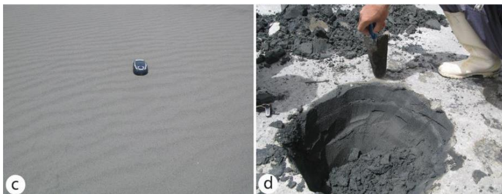
ادامه شکل ۱. (c) ریپل‌مارک‌های بادی در سواحل ماسه‌ای؛ (d) تصویری از لایه‌های ماسه‌ای سیاه‌رنگ در بستر ساحل غربی دریاچه ارومیه
