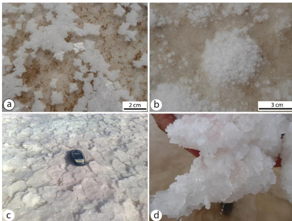
شکل ۵. a) رشد کانی هالیت به صورت بلورهای کوبیک اسکلتی هوپر؛ b) رشد بلورهای کوبیک هالیت و ایجاد ساخت های گل کلمی در بستر دریاچه؛ c) رشد بلورهای ورقه ای هالیت؛ d) بلورهای هگزائوکتاهندرال درشت و شفاف سیلویت.
